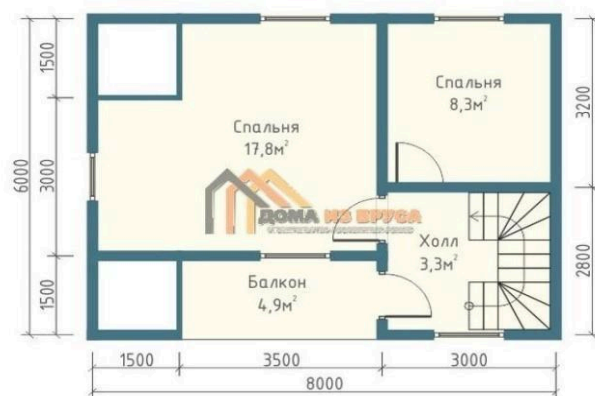
План 2-го этажа
