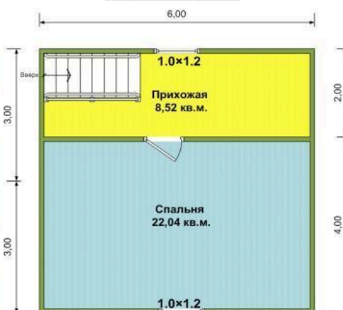
План 2-й этаж
