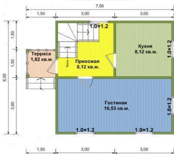
План 1-й этаж
